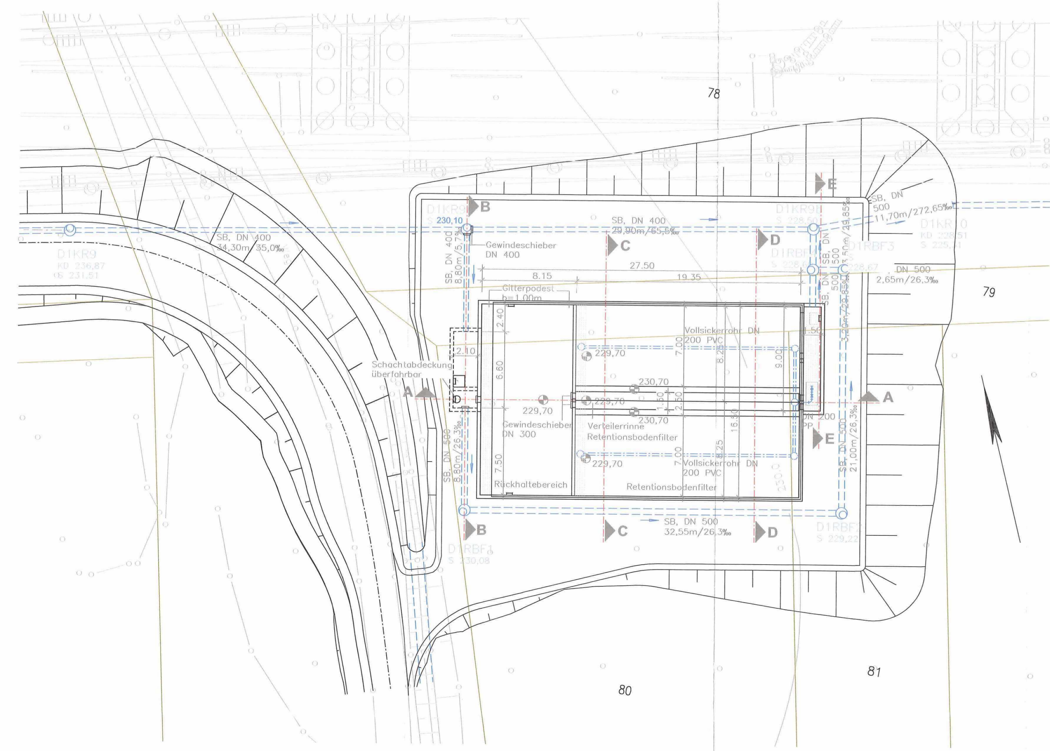
Draufsicht Retentionsfilterbecken 1 Maßstab 1:200
