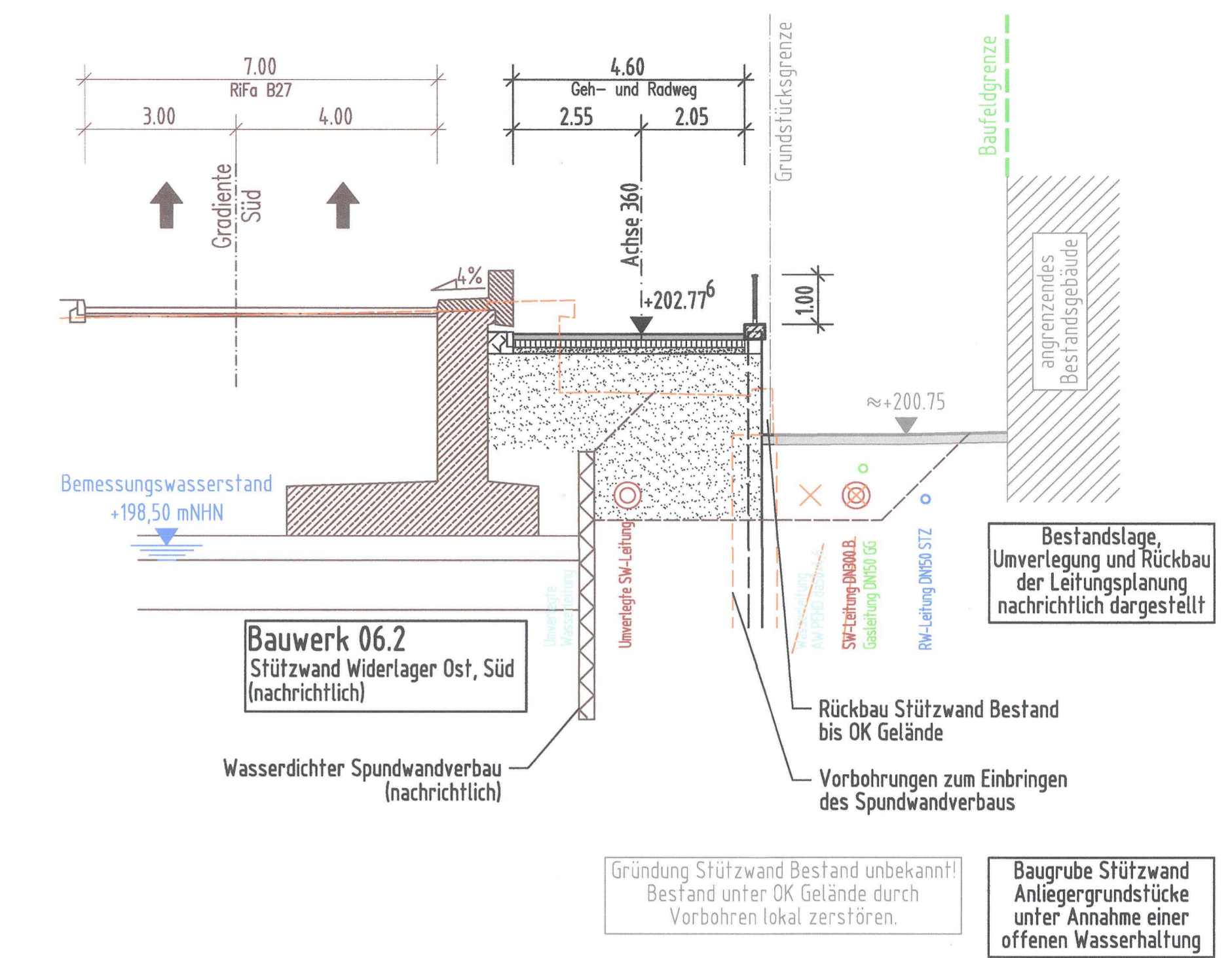
Schnitt B-B M. 1:100 Querschnitt Stützwand Anliegergrundstücke und Rampe Industriestraße
