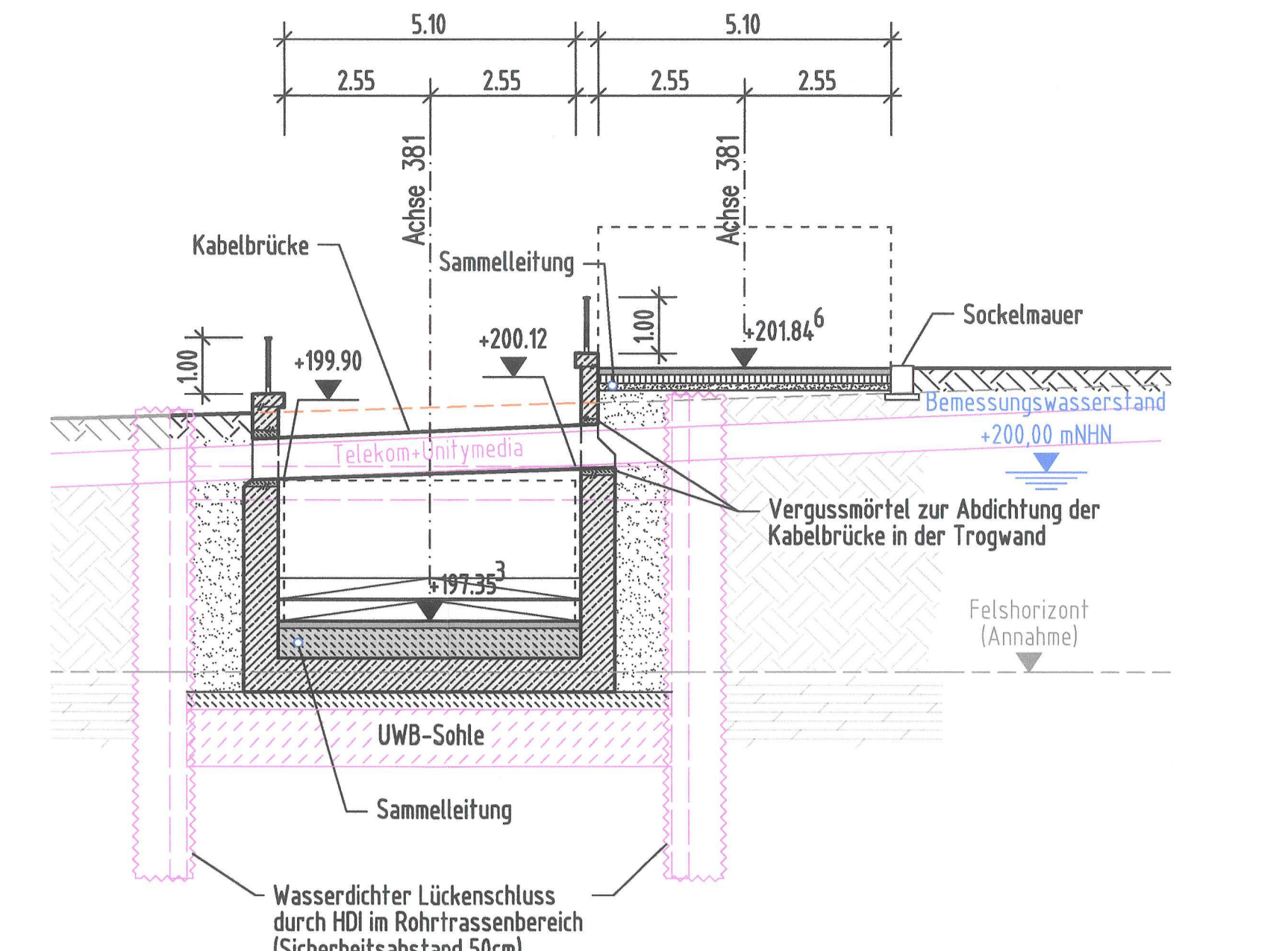
Schnitt B-B M. 1:100 Kabelbrücke und Querschnitt Rampe FU West
