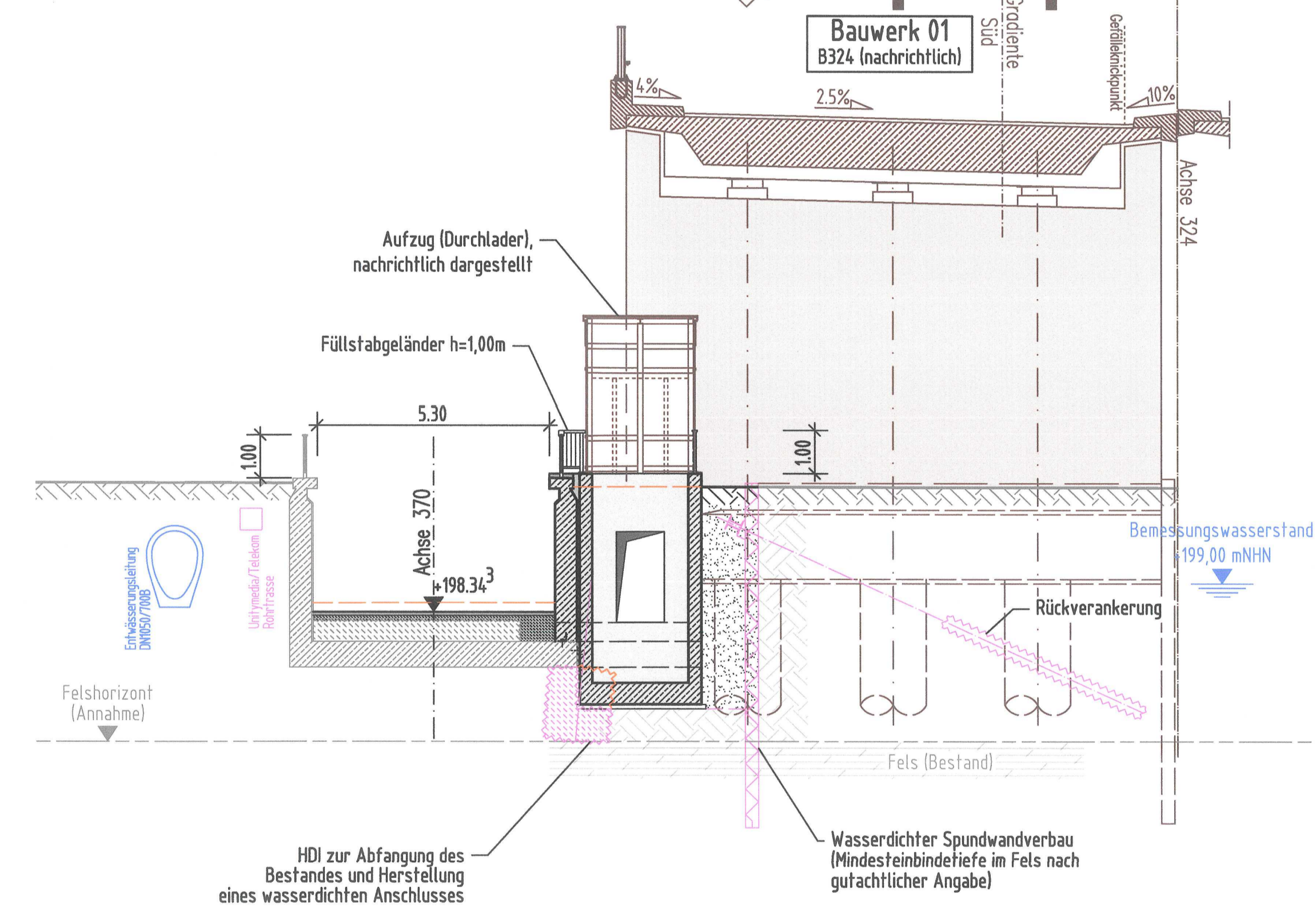
Schnitt C-C M. 1:100 Querschnitt Rampe und Aufzugschacht
