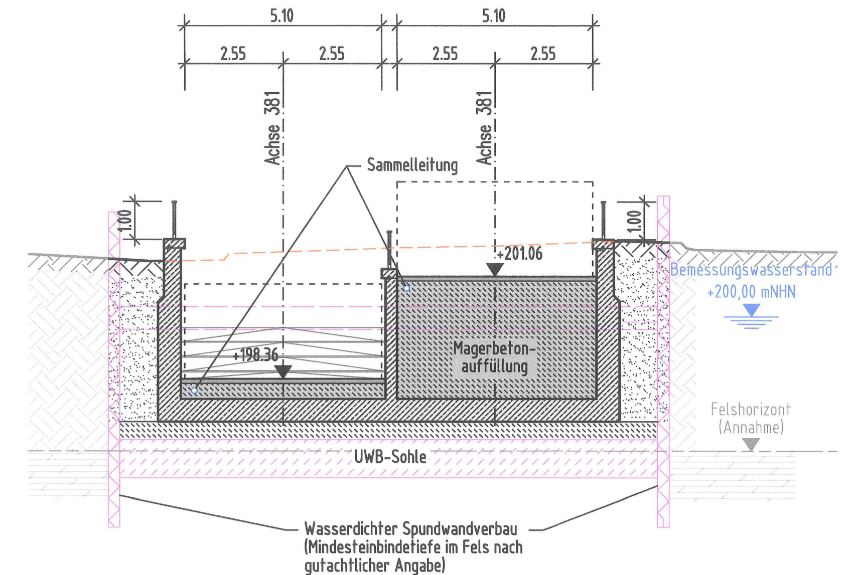
Schnitt A-A M. 1:100 Querschnitt Rampe FU West
