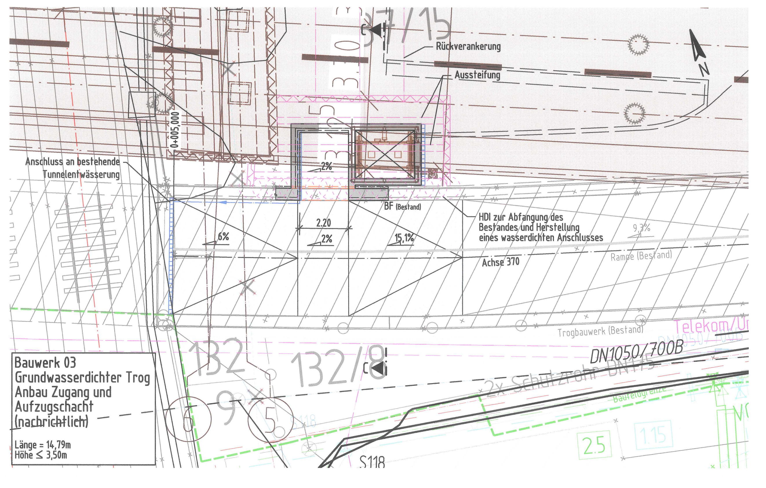
Draufsicht Rampe Fußgängerunterführung Ost M. 1:100
