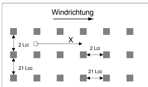
Bild 3: Ausbreitung in ebenem Gelände mit gleichförmiger Bebauung
